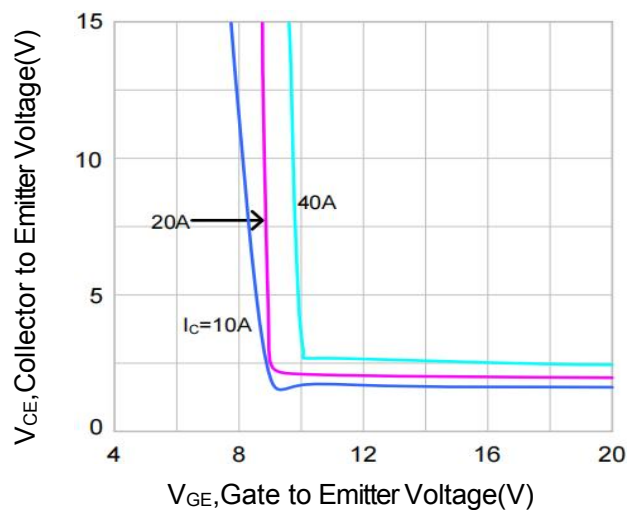
Fig 6. V_{CE(sat)} vs. V_{GE}(V)
